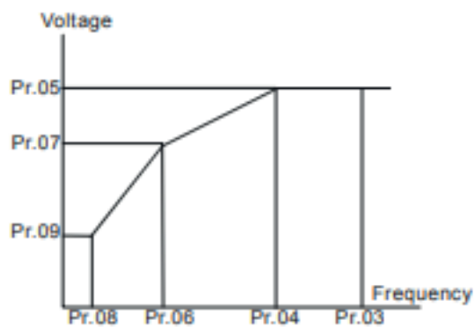
منحنی V/F دلخواه
