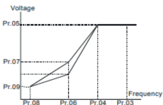
منحنی V/F فن و پمپ
