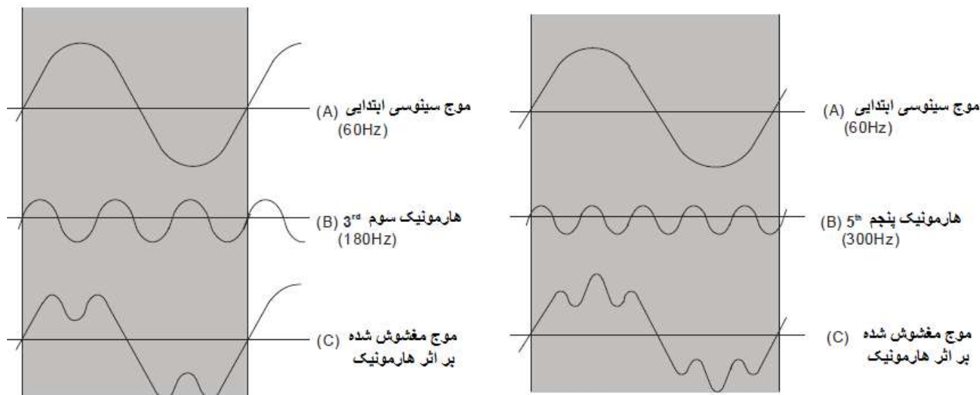
تاثیر هارمونیک سوم و پنجم بر موج سینوسی جریان
