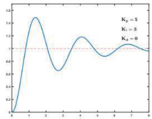
پاسخ سیستم با کنترلر PI
