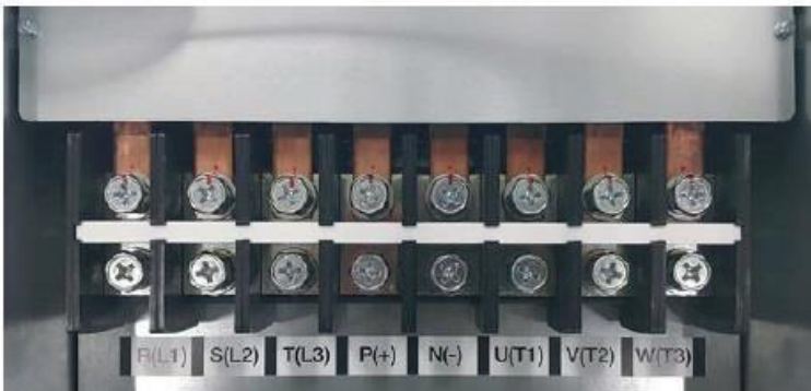
Power terminal (F3~F6)
