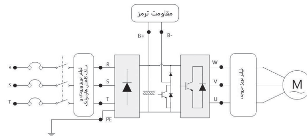
شکل ۷ الف نمایش ترمینال‌های قدرت ورودی و خروجی درایو سه فاز
