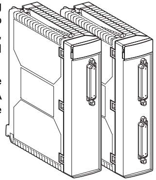
TSX AEY 800 / AEY 1600
