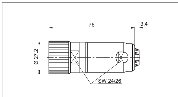
Fan plug
